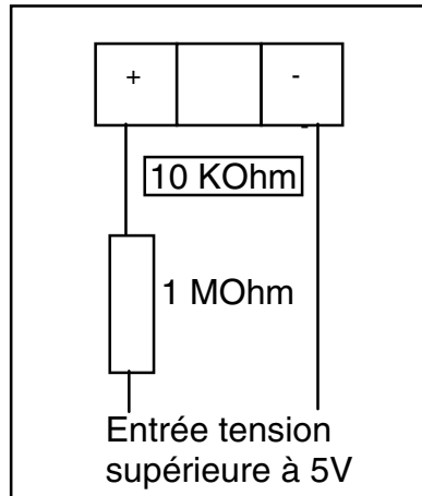
Connexion d'une entrée > 5V
